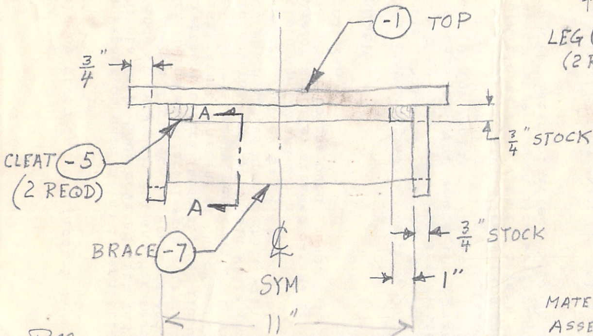
STEP STOOL
